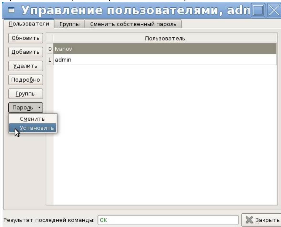
Рисунок 3.18 – Установка пароля
